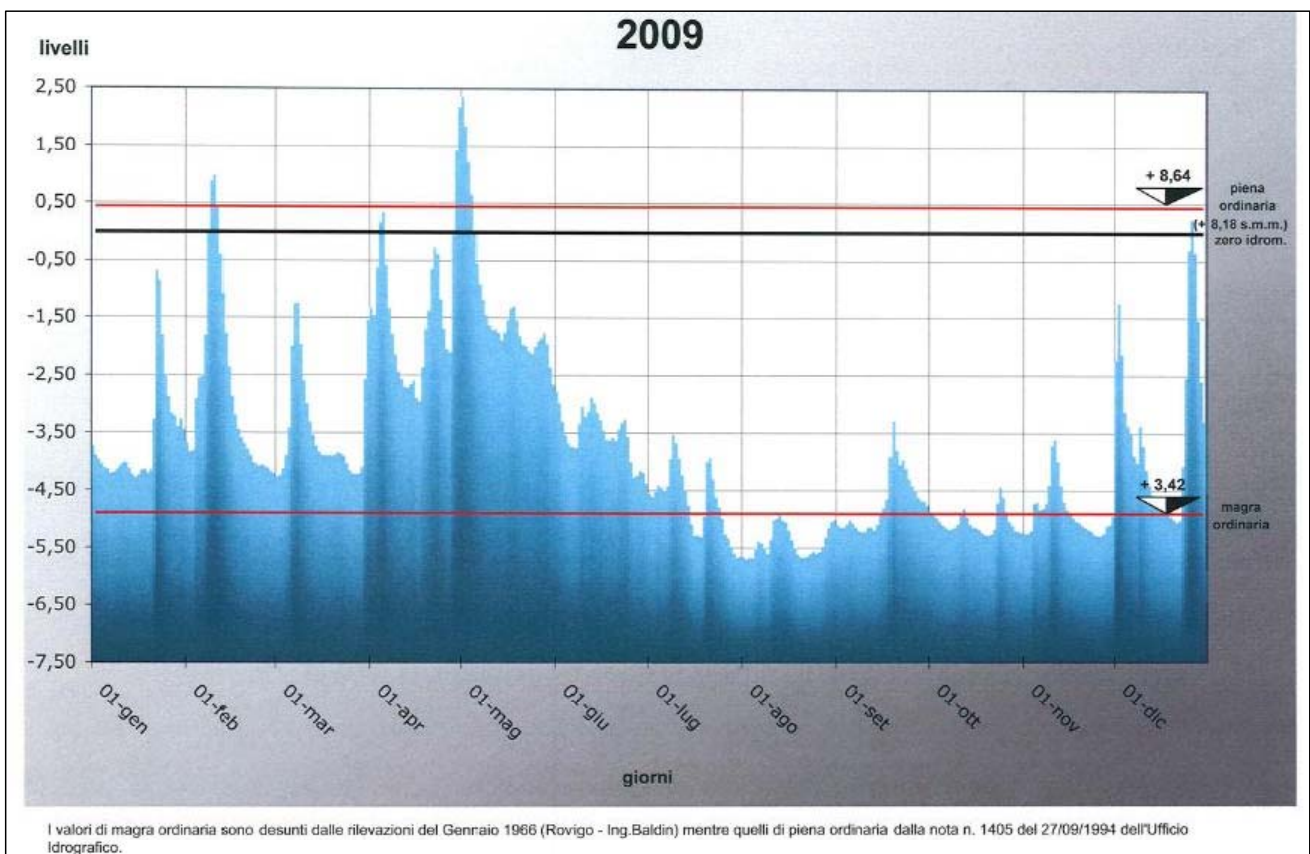
Graf. 1.39 - Livelli idrometrici giornalieri del fiume Po (m. rispetto allo zero idrometrico), rilevati alle ore 8.00 presso l'idrometro di Pontelagoscuro per l'anno 2009
