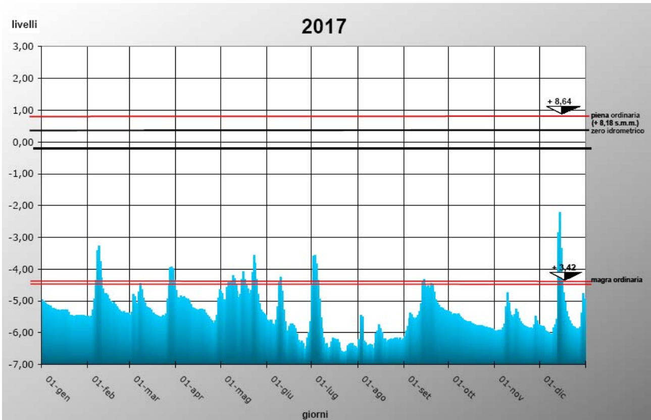
Graf. 1.20 - Livelli idrometrici giornalieri del fiume Po (m. rispetto allo zero idrometrico), rilevati alle ore 8.00 presso l'idrometro di Pontelagoscuro per l'anno 2017
